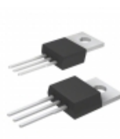
DSEC29-02A IXYS DIODE ARRAY GP 200V 15A TO220AB
