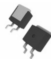
DSEC29-02AS IXYS DIODE ARRAY GP 200V 15A TO263
