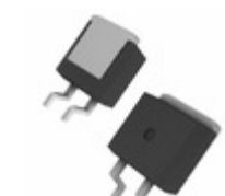
DGS10-025AS IXYS DIODE SCHOTTKY 250V 12A TO263AB
