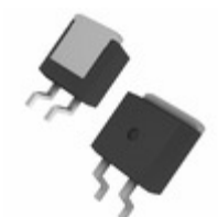
IXFA16N50P3 IXYS MOSFET N-CH 500V 16A TO-263AA
