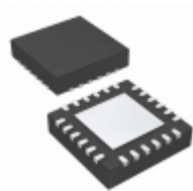
PCA9675BQ,118 NXP USA Inc. IC I/O EXPANDER I2C 16B 24DHVQFN
